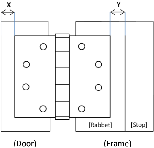
HINGE BACKSETS
