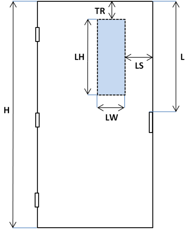
DOOR HANDING
